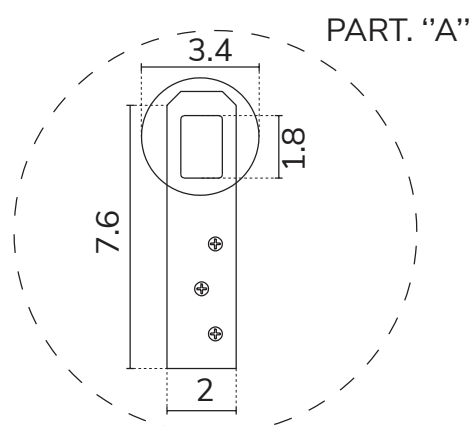
PARTICOLARE MONTAGGIO FISCHER / detail fitting fischer
