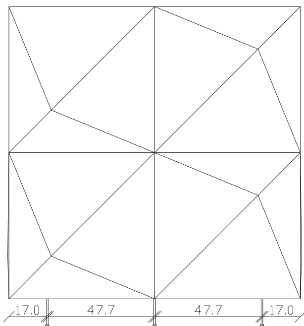
BASE (vista dal basso)
